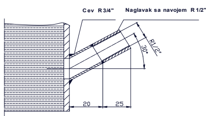
Skica ugradnje elektroprovodne sonde
